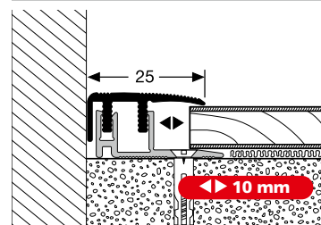
PF 587 L Maxx ⬆ 8 - 12 mm
