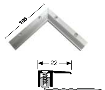
PF 487 IE \varnothing 7-15 mm 90° Innenecke 90° Inner Corner 90° Angle Intérieur
