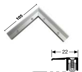
PF 487 AE \varnothing 7-15 mm 90° Außenecke 90° Outer Corner 90° Angle Extérieur
