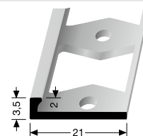
PF 299 G \pm 2 mm geschlossen gestanzt punched base estampé fermé
